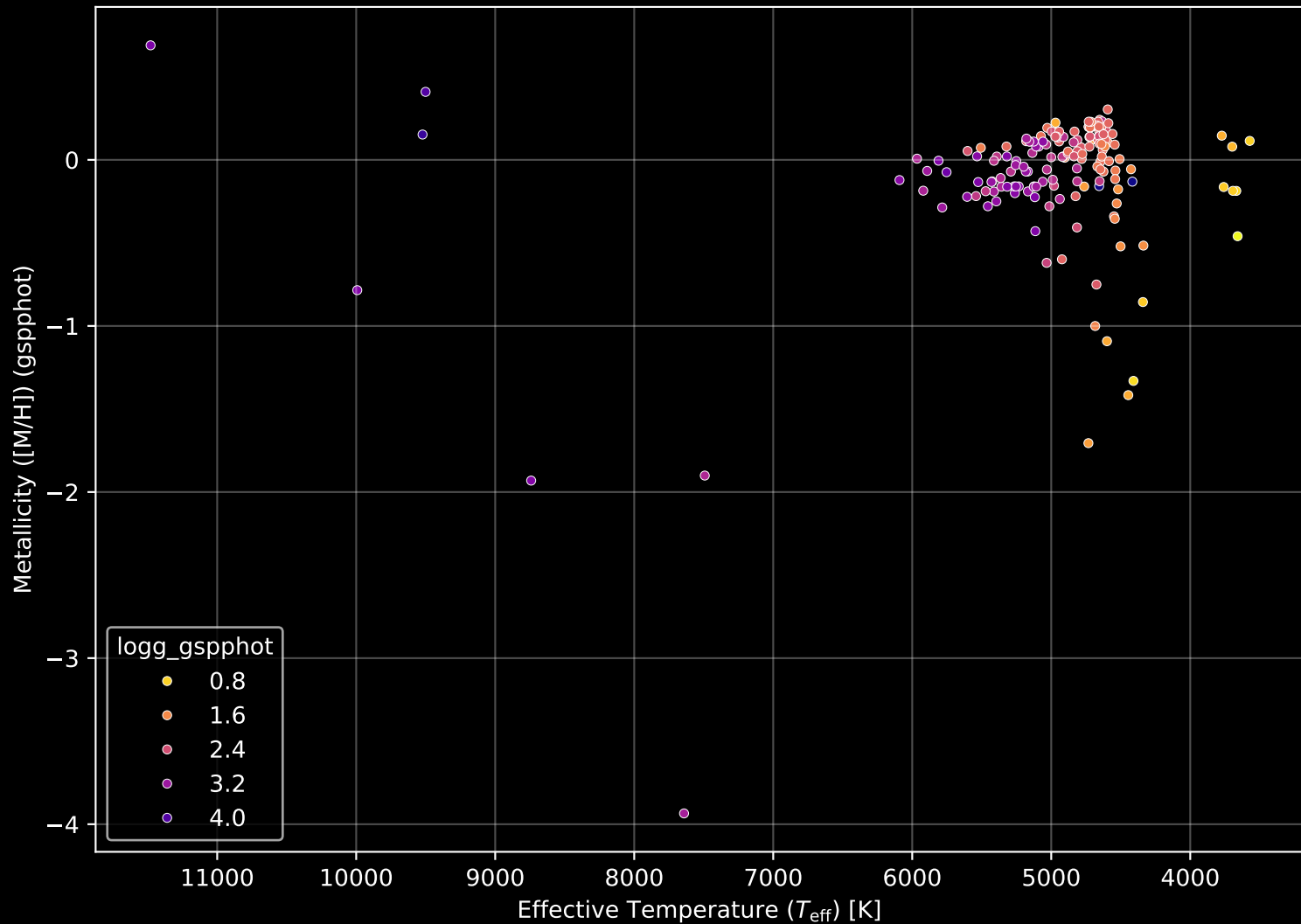
APOGEE DR17 Field: [Berkeley_18_btx] Stellar Population Parameters (n= 168)
